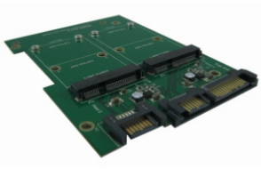
AD963DE9 转接卡
